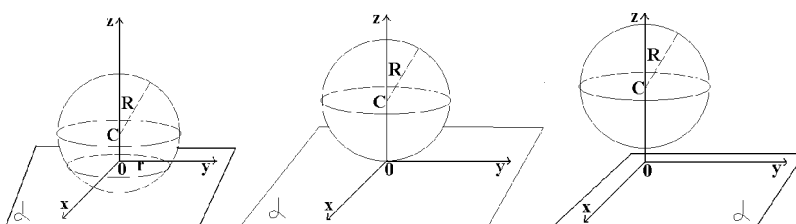
Рисунок 66. Взаимное расположение сферы и плоскости
