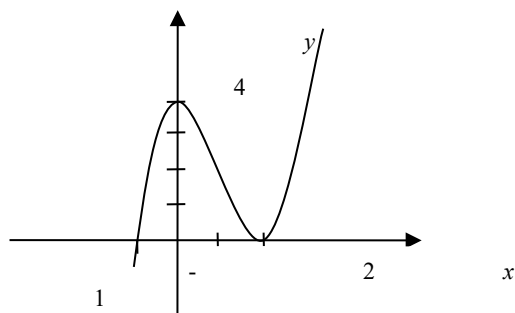
Рисунок 23. График функции y=(x+1) \cdot (x-2)^2
